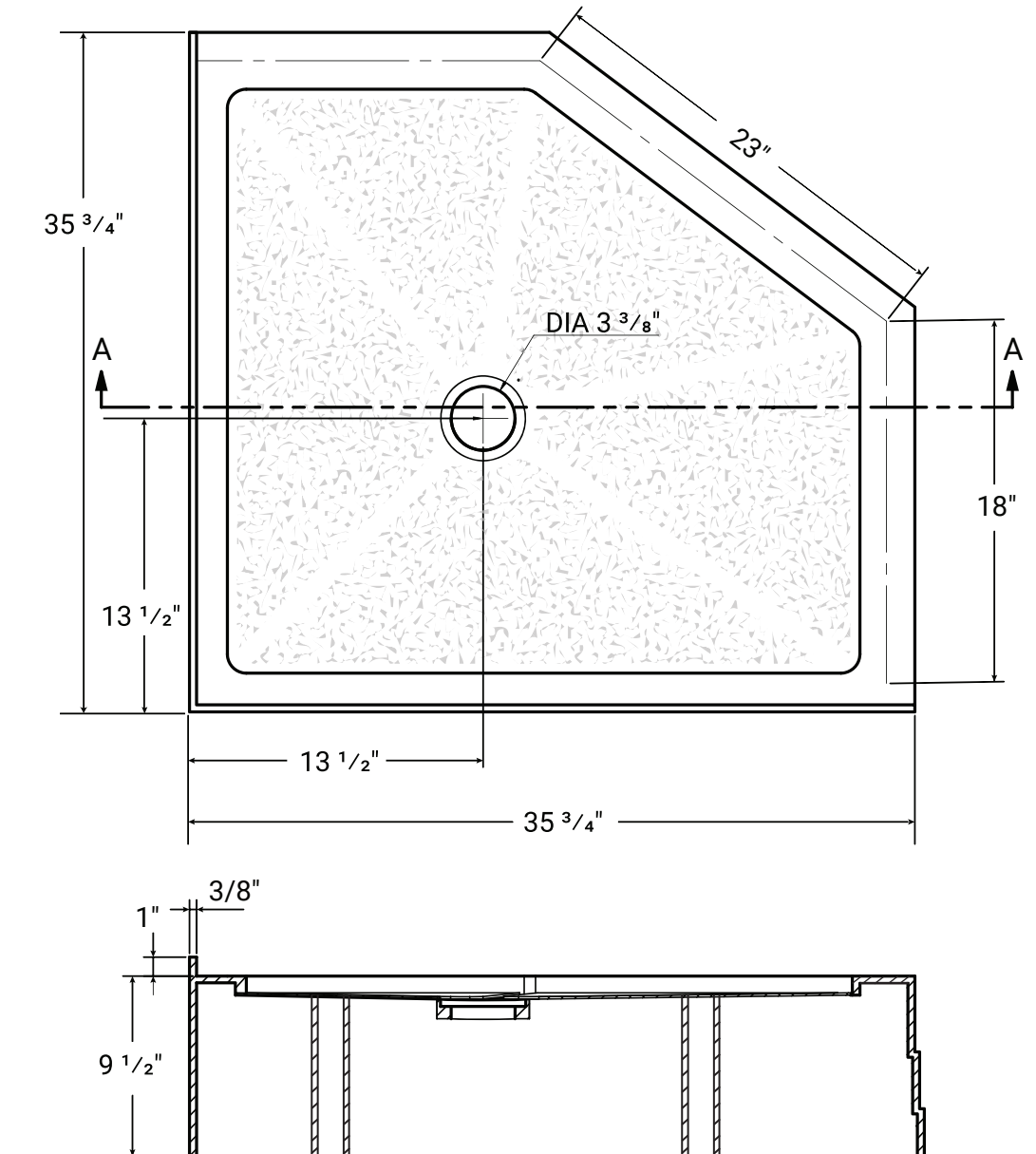
SECTION A-A
